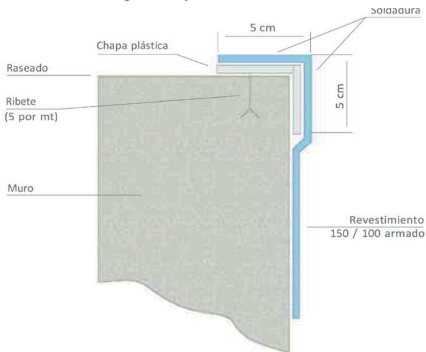
Figura 3A: Fijación sobre raseado
