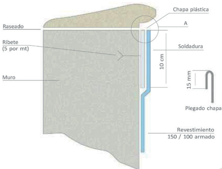
Figura 3B: Fijación sobre pared vertical (renovación)
