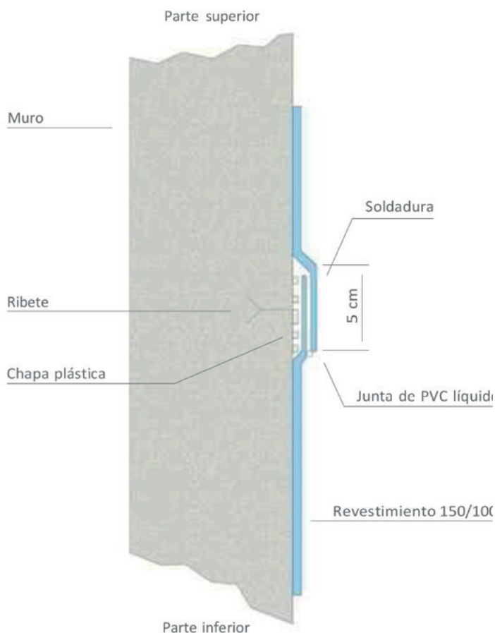
Figura 6: Fijación mecánica intermedia pared plana
